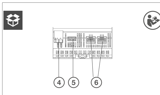
Afbeelding 4: Ontwerp en lay-out van het apparaat - onderaanzicht op KNX-, USB- en Ethernet-interfaces
