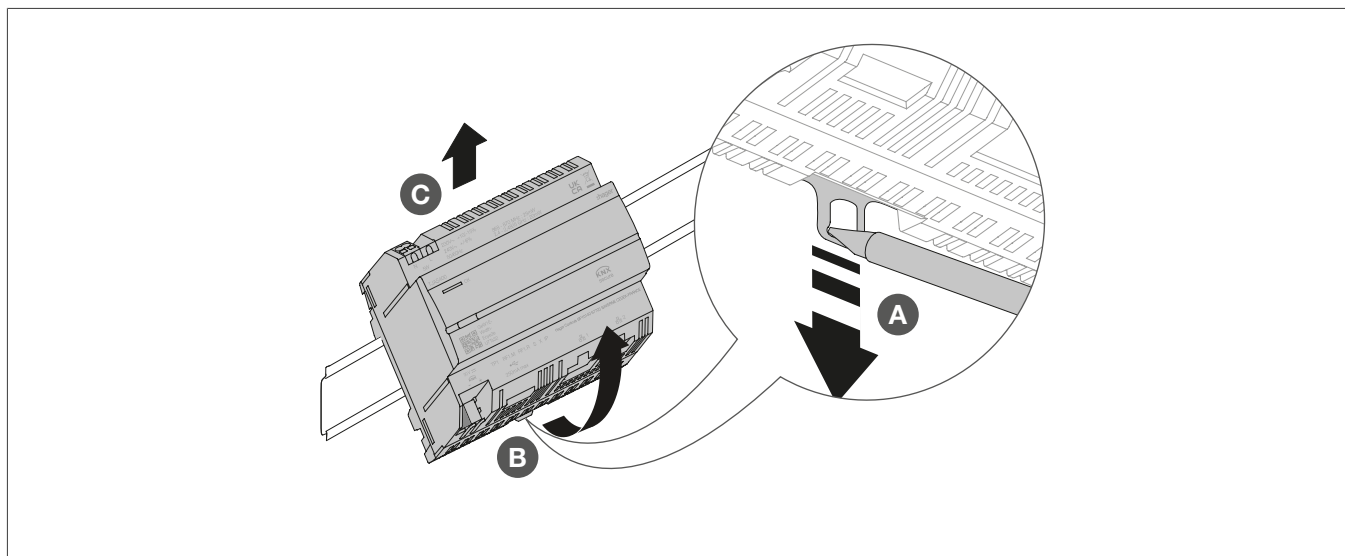
Afbeelding 17: Het apparaat van de DIN-rail verwijderen
