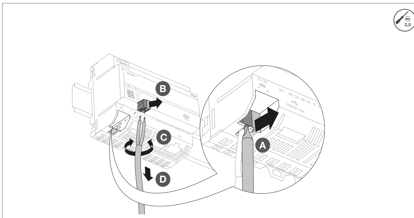
Afbeelding 15: De busverbindingsklemmen verwijderen
