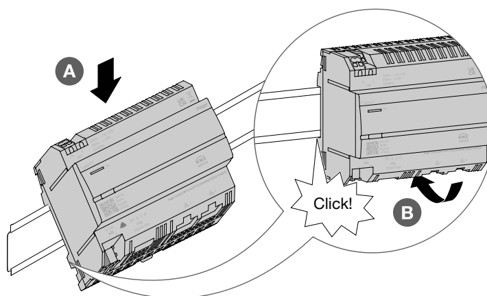
Afbeelding 9: Het apparaat op de DIN-rail monteren
