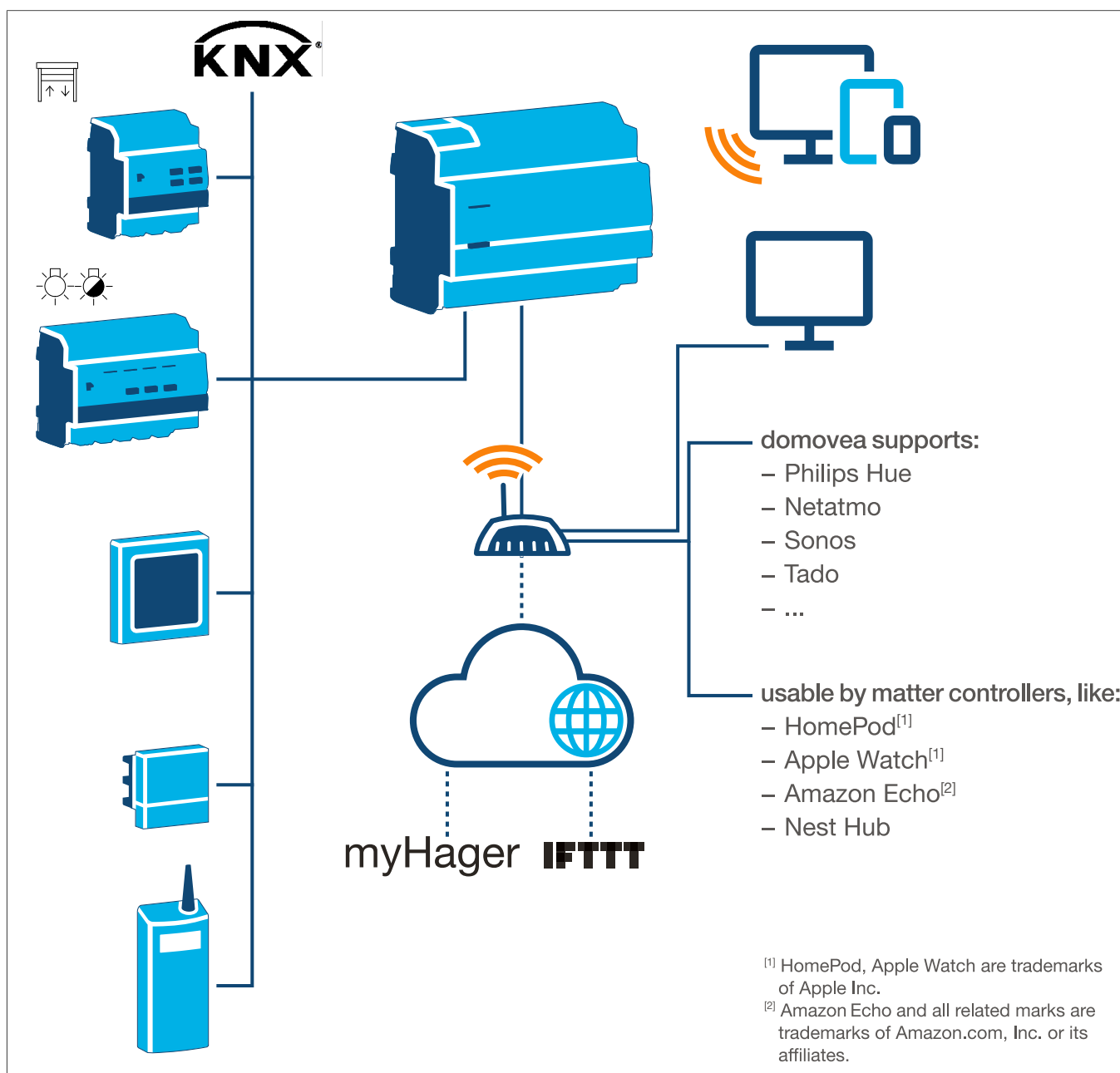
Afbeelding 7: Overzicht installatie
