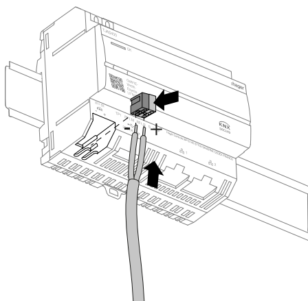
Afbeelding 13: De buskabel aansluiten
