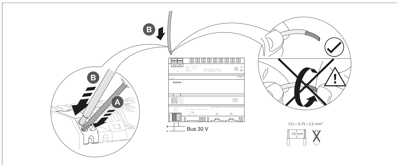
Afbeelding 11: Het apparaat aansluiten
